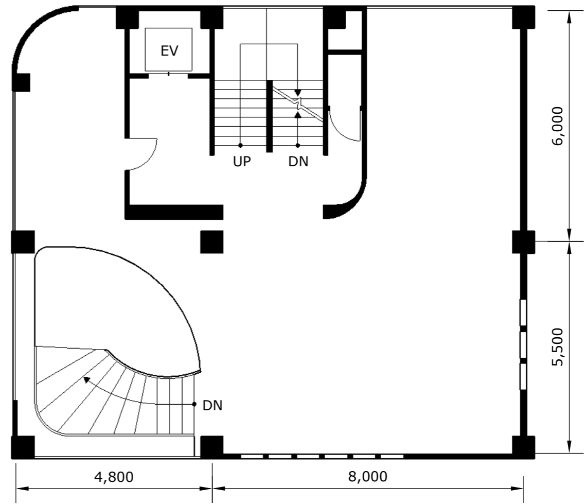
3、4階 平面図 1/100
