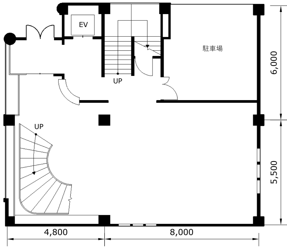
1階 平面図 1/100
