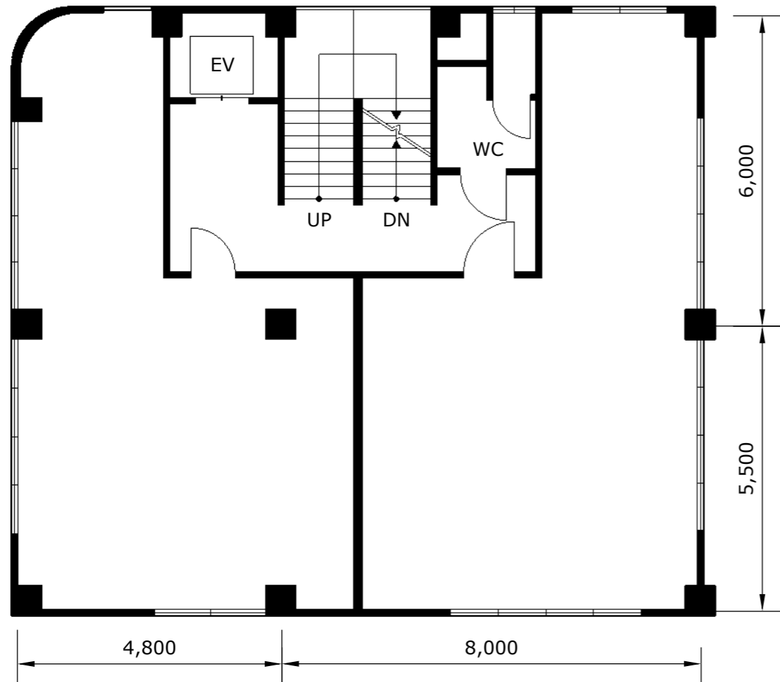
2階 平面図 1/100
