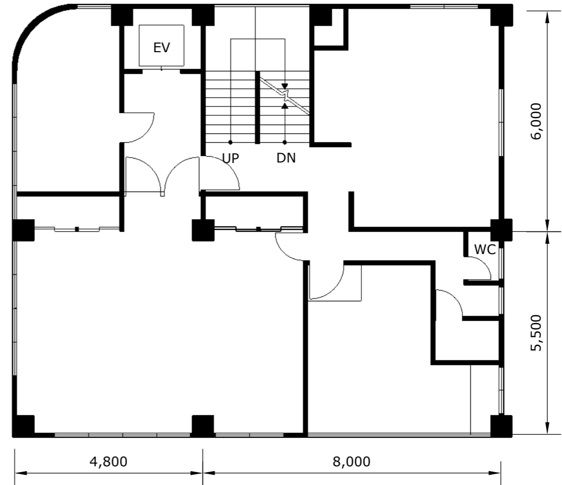
5階 平面図 1/100
